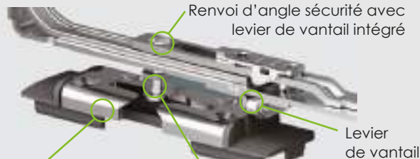
Renvoi d'angle sécurisé en partie haute
